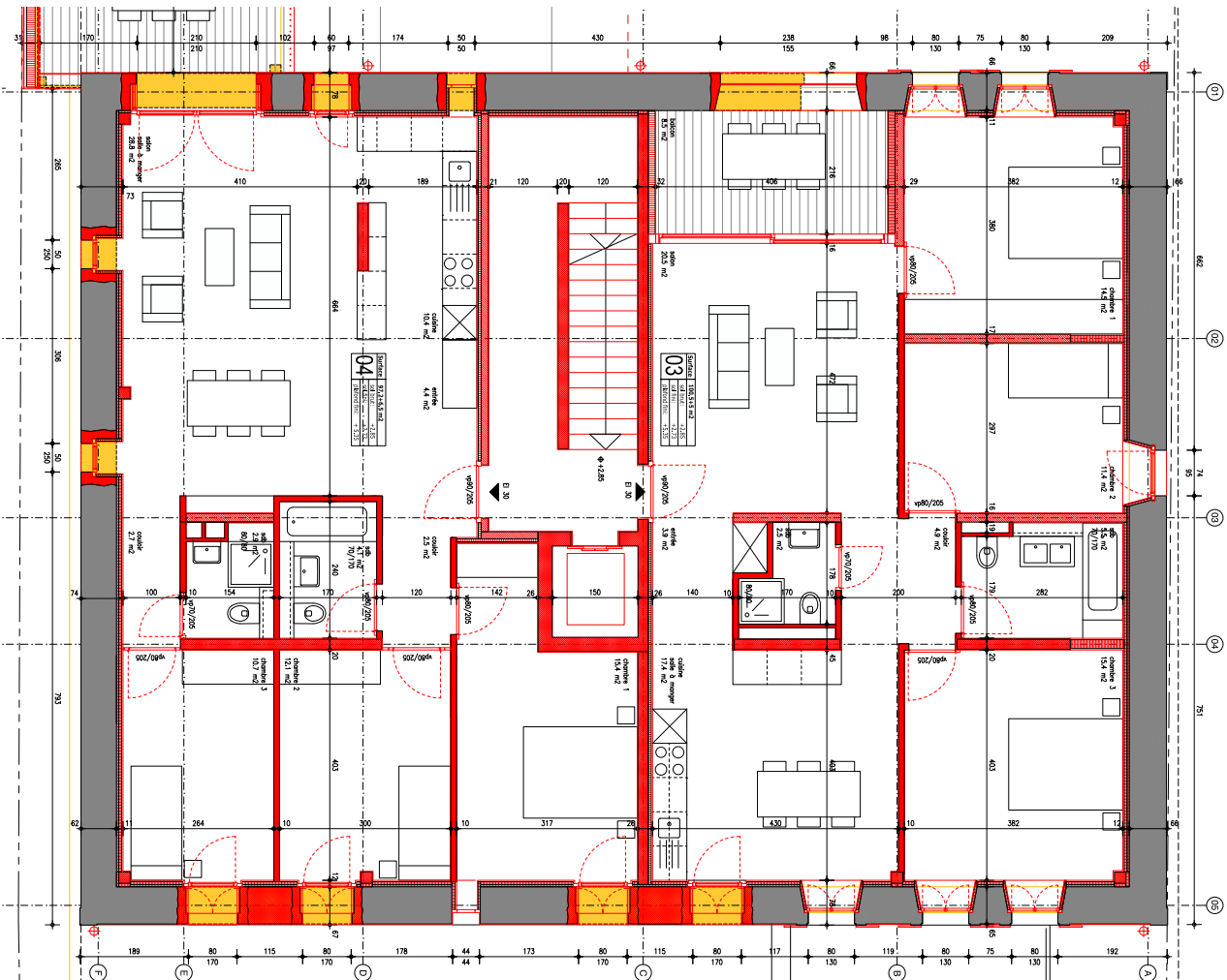
plan niveau 1
